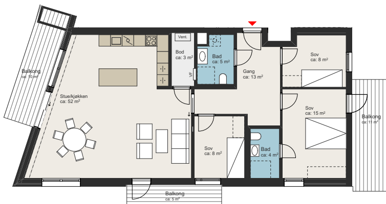
A-401, 501, 601 BRA 114 m 2
