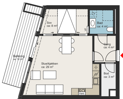
A-402, 502, 602 BRA 51 m 2
